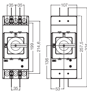
Tamaño 400 3P + MRI DWB400
