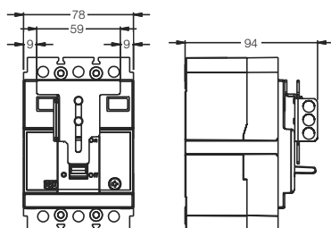
Tamaño 160 3P + PLW DWB160 3P
