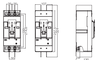
Tamaño 400 3P + PLW DWB400
