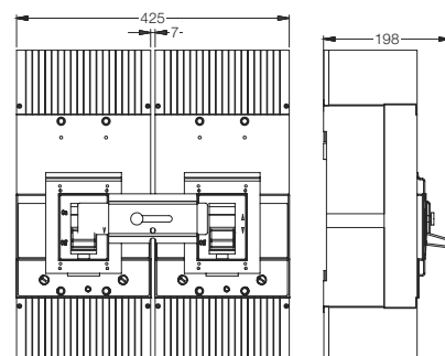
Tamaño 1600 3P + BLIM DWA800-1600
