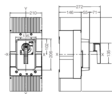
Tamaño 1600 3P + MRI DWA1600
