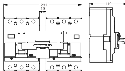
Tamaño 250 3P + BLIM DWB250 3P
